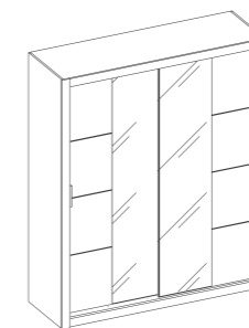
ID-03 szafa z drzwiami przesuwными, drążkiem i półkami 180 x 215 x 60 cm
