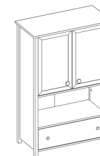
LN-11 komoda z szufladą 85 x 131 x 42 cm
