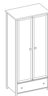
SO-12 szafa z drążkami, półkami i szufladą 85 x 186 x 52 cm
